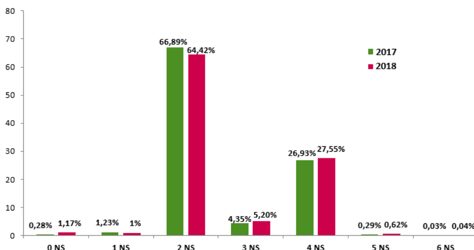
Figure 16: Nombre de serveurs NS par nom de domaine .ma
