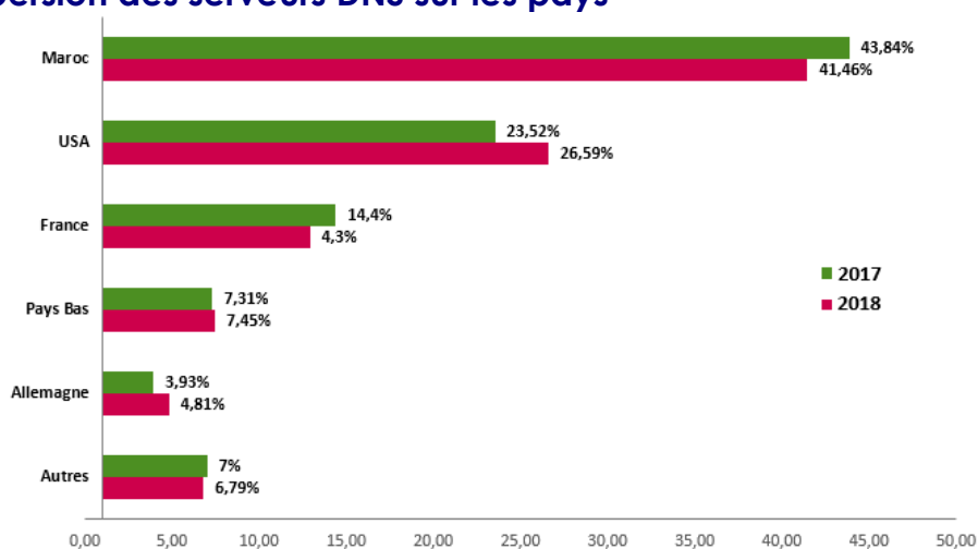
Figure 17: Dispersion des serveurs DNS sur les pays
