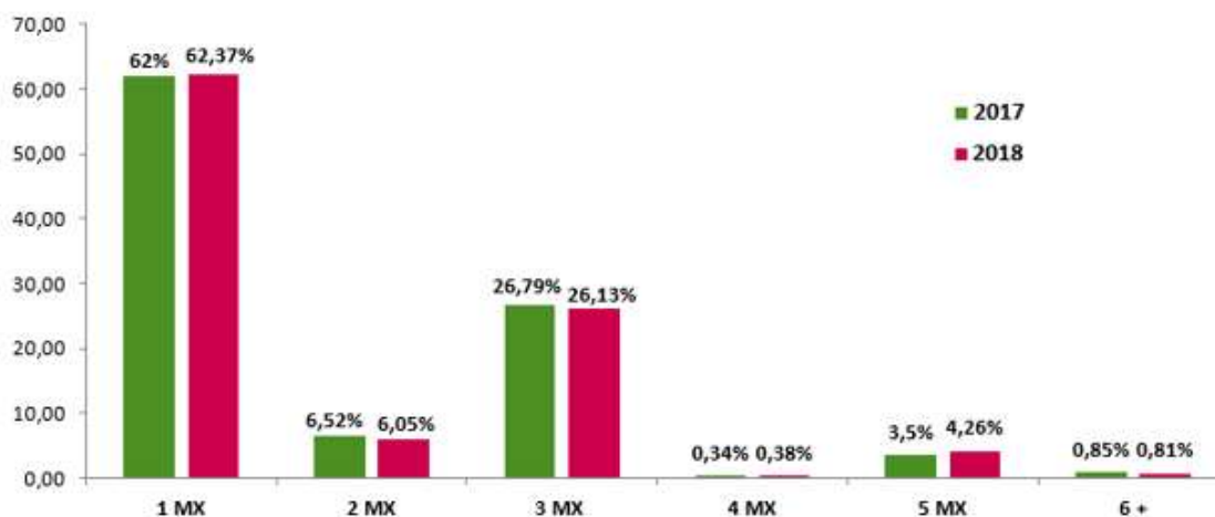
Figure 19: Nombre de relais par nom de domaine .ma
