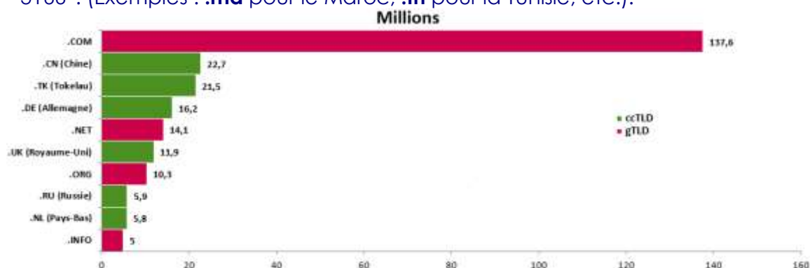
Figure 1: Nombre de noms de domaine dans le Monde à fin septembre 2018
